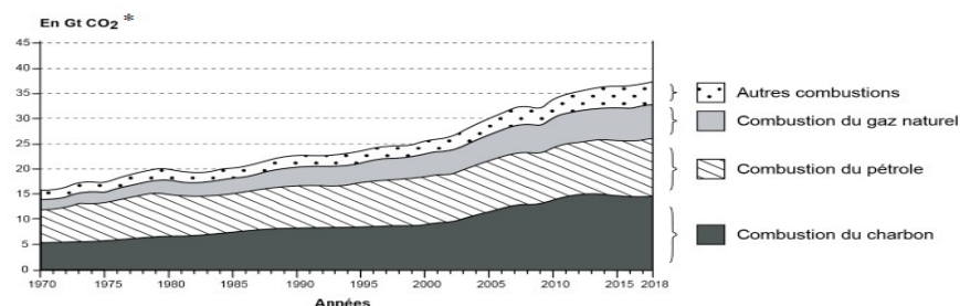
Émissions annuelles de CO 2 par combustible dans le monde
